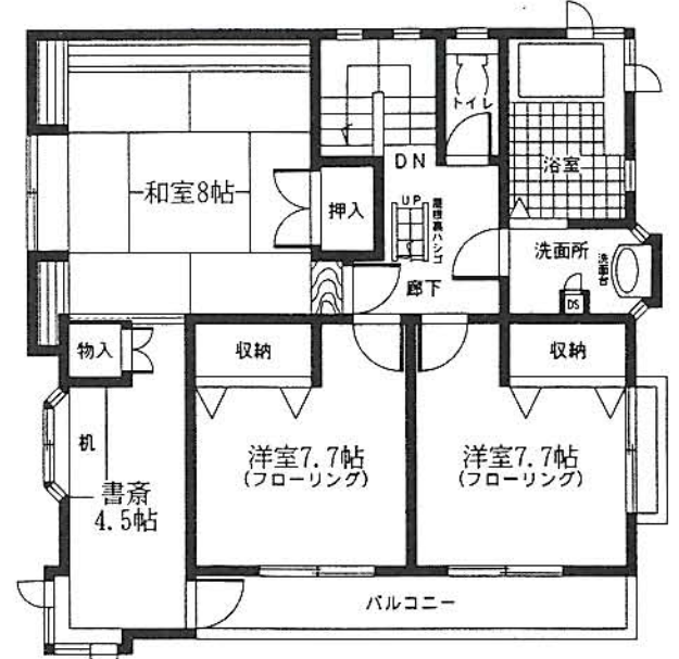
【2階平面図】
