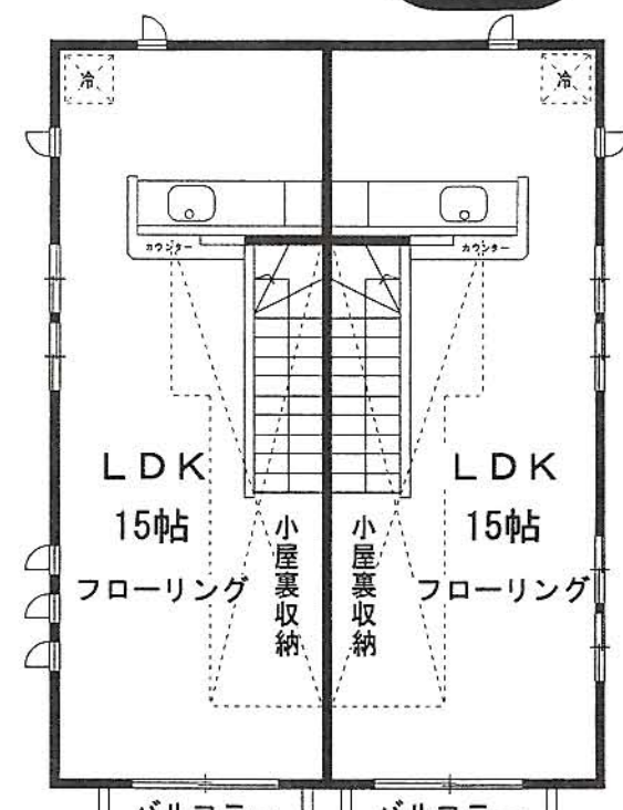
2階 【E号室2階】 【W号室2階】
