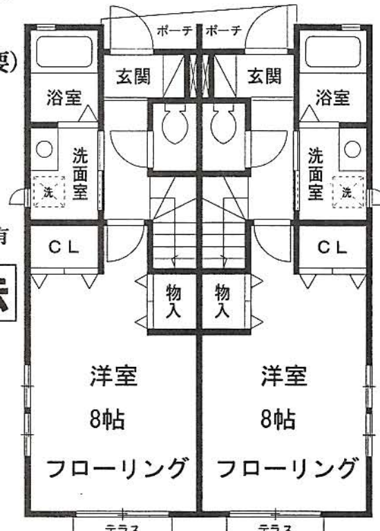
1階 【E号室1階】 【W号室1階】
